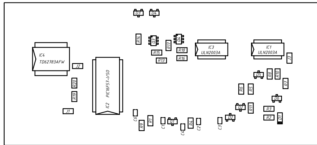
Плата БК-100 Сборочный чертеж
