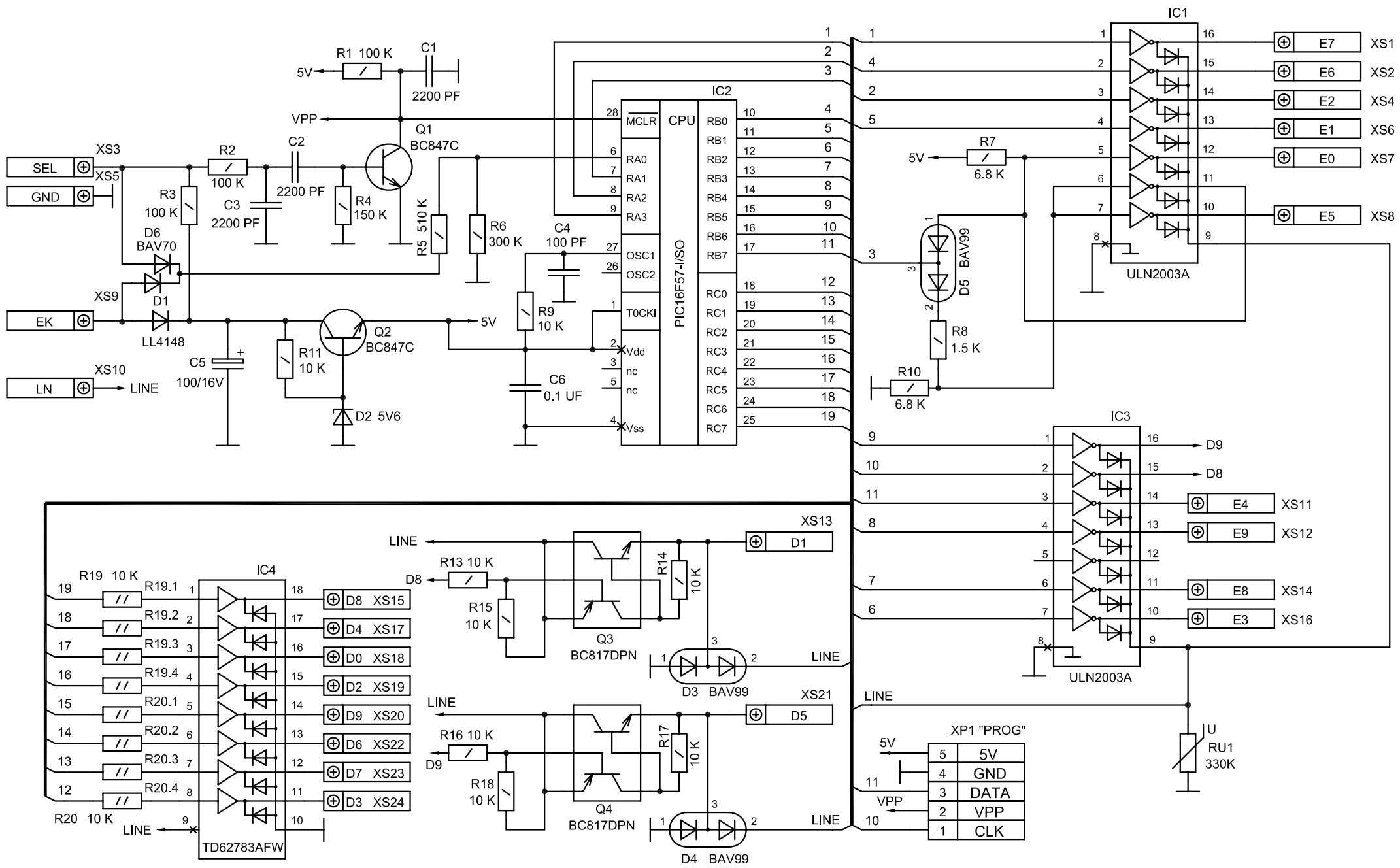
Блок коммутации БК-100 Схема электрическая принципиальная
