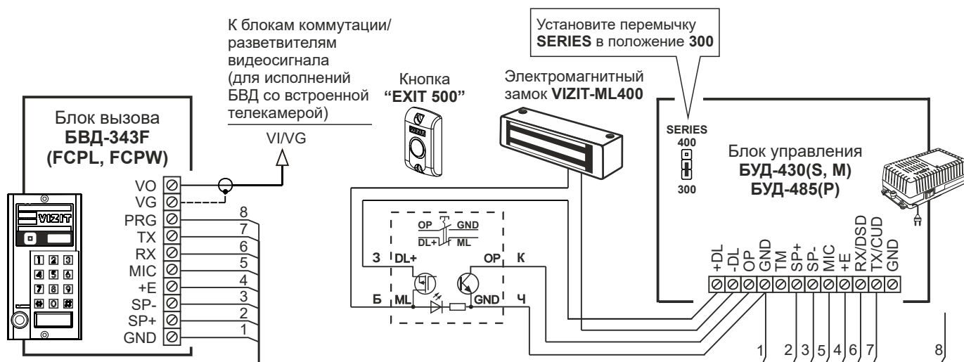
Рисунок 10 - Схема соединений блока вызова БВД-343F(FCPL, FCPW) с блоком управления БУД-430(S, М), БУД-485(Р) , электромагнитным замком VIZIT-ML400 и кнопкой “EXIT 500”
