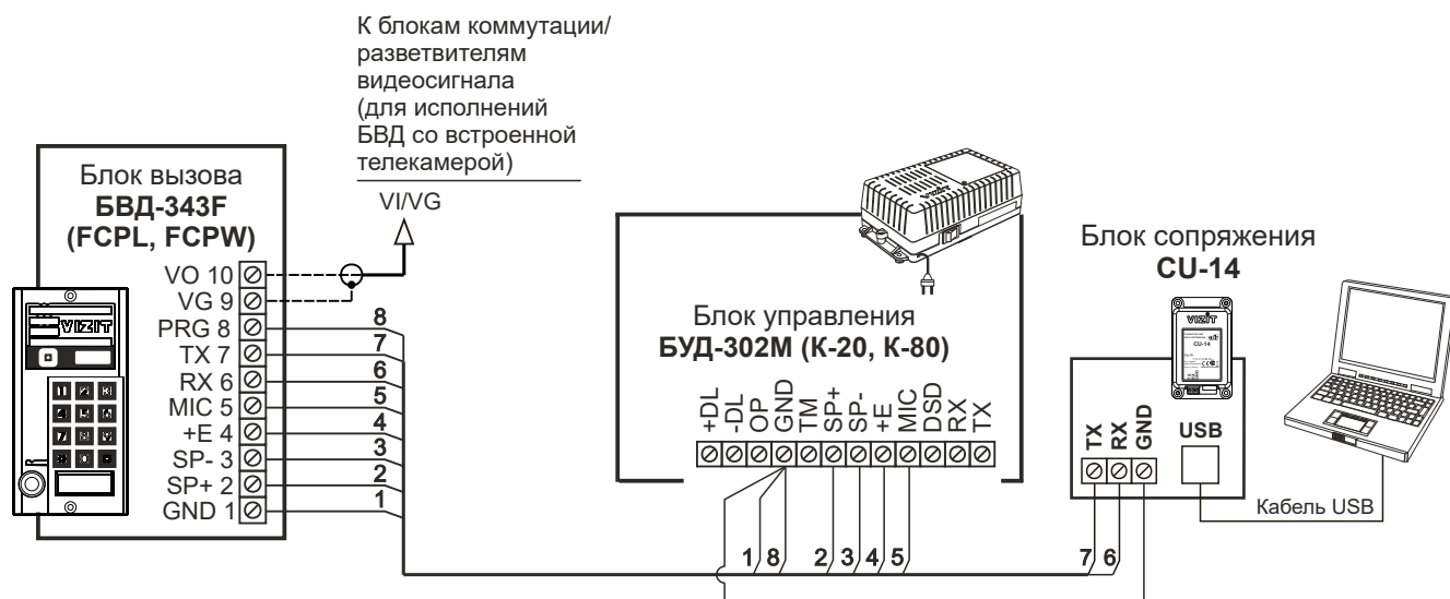
Рисунок 12 - Схема соединений блока вызова с блоками управления БУД-302М(К-20, К-80) и блоком сопряжения CU-14
