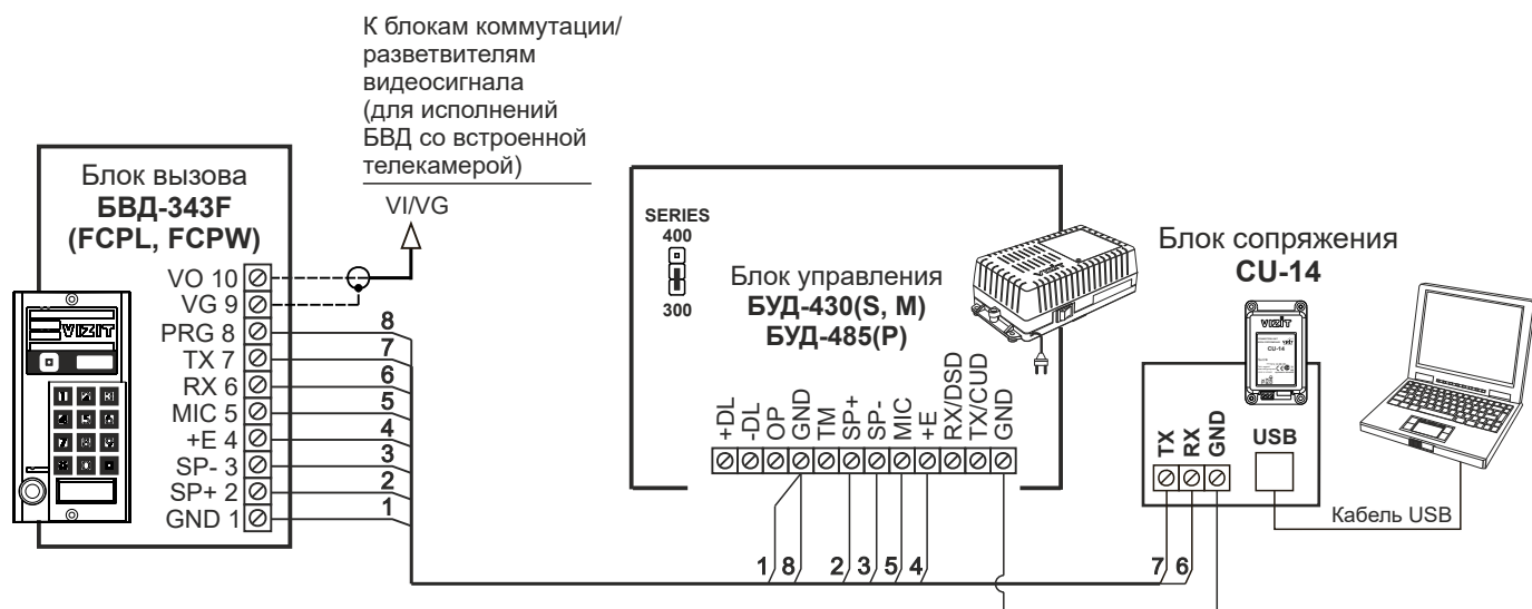
Рисунок 13 - Схема соединений блока вызова с блоками управления БУД-430(С, М), БУД-485(Р) и блоком сопряжения CU-14
