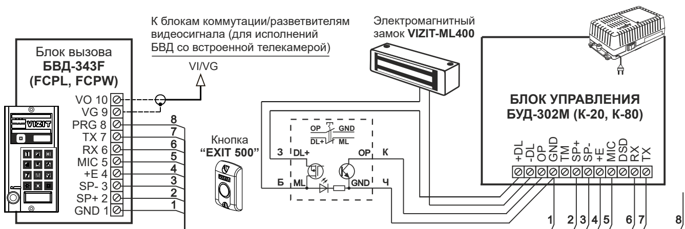
Рисунок 7 - Схема соединений блока вызова БВД-343F(FCPL, FCPW) с блоком управления БУД-302М (К-20, К-80), электромагнитным замком VIZIT-ML400 и кнопкой "EXIT 500"
