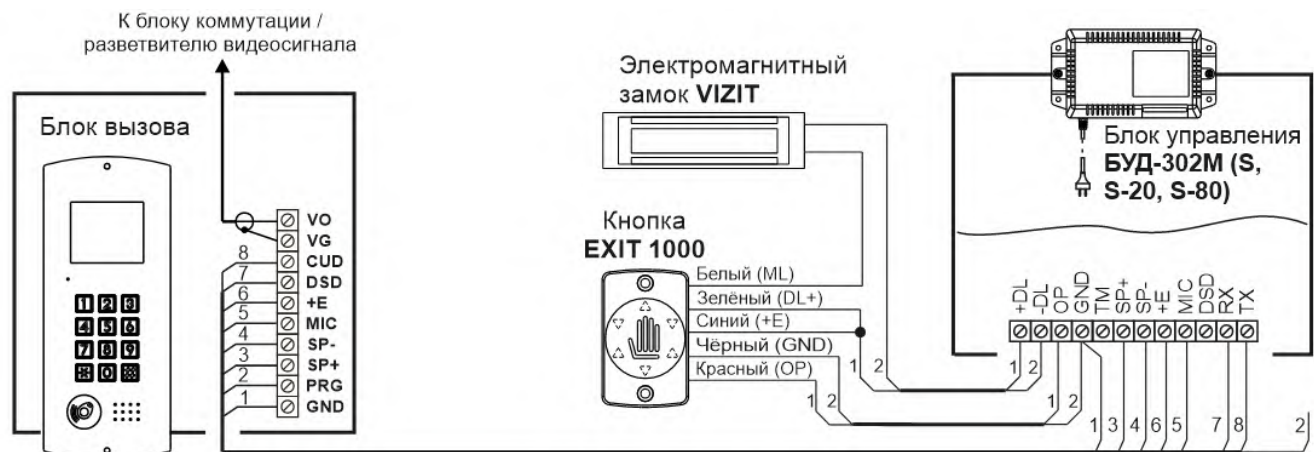
Рисунок 8.4 – Схема соединений блока вызова с блоком управления БУД-430(M,S), -480(S), -485(M,P) и электромеханическим замком / защёлкой
