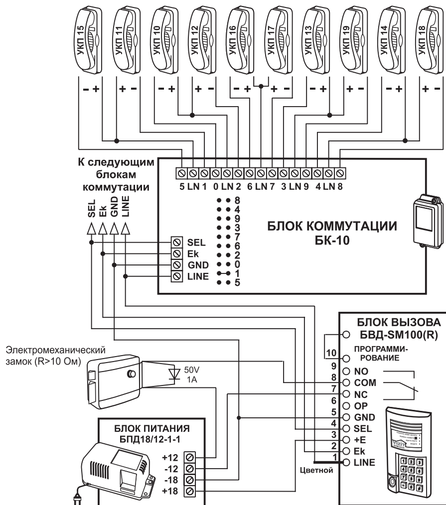
Рисунок 3 - Схема соединений блоков домофона с использованием блоков коммутации БК-10
