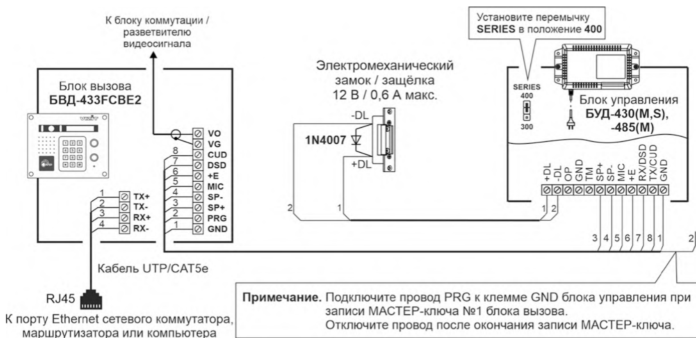
Рисунок 8.3 – Схема соединений блока вызова с блоком управления БУД-430(М,С), -480(С), -485(М), электромагнитным замком VIZIT и кнопкой EXIT 300M
