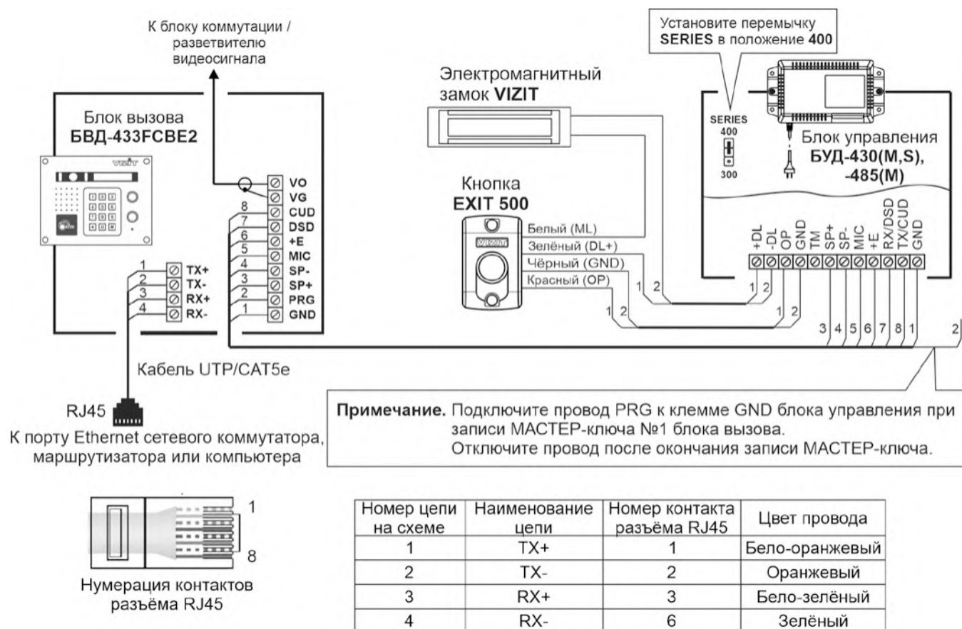
Рисунок 8.2 – Схема соединений блока вызова с блоком управления БУД-430(М,С), -480(С), -485(М,MP), электромагнитным замком VIZIT и кнопкой EXIT 500
