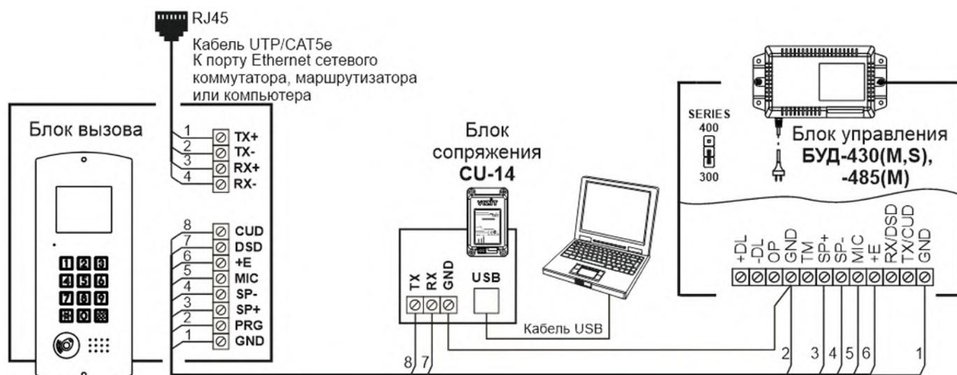
Рисунок 16.1 - Схема соединений блока вызова с блоками управления БУД-430(S, M), -430(S), -485(M) и блоком сопряжения CU-14
