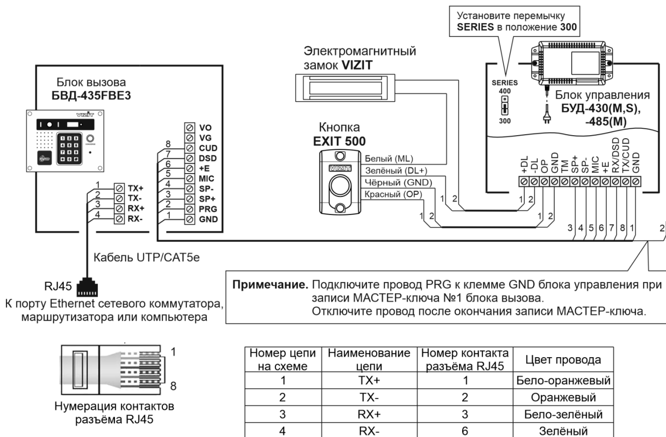
Рисунок 8.2 – Схема соединений блока вызова с блоком управления БУД-430(М,С), -485(М,Р), электромагнитным замком VIZIT-ML400 и кнопкой EXIT 500
