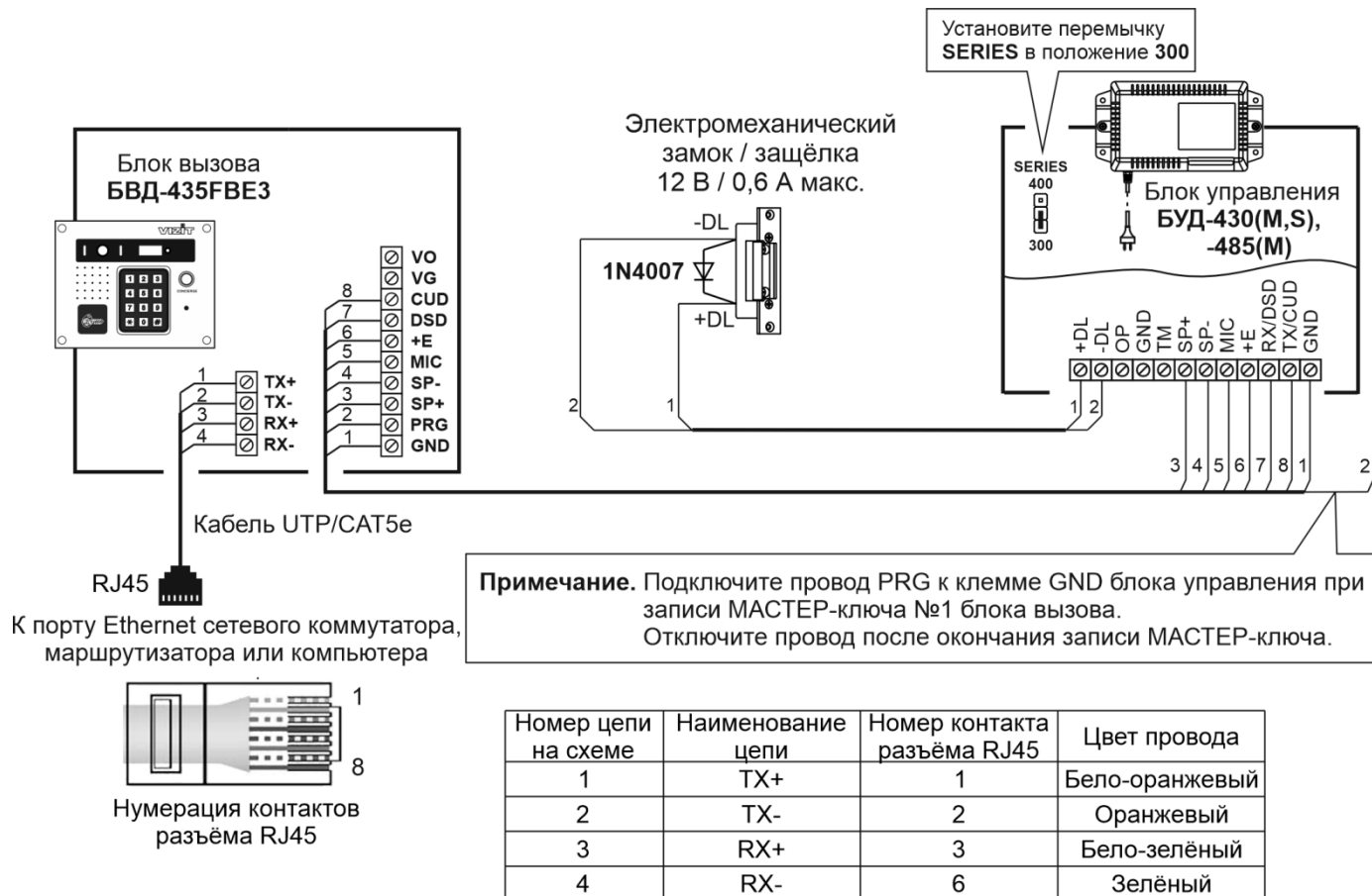
Рисунок 8.4 – Схема соединений блока вызова с блоком управления БУД-430(М,С), -485(М,Р) и электромеханическим замком / защёлкой
