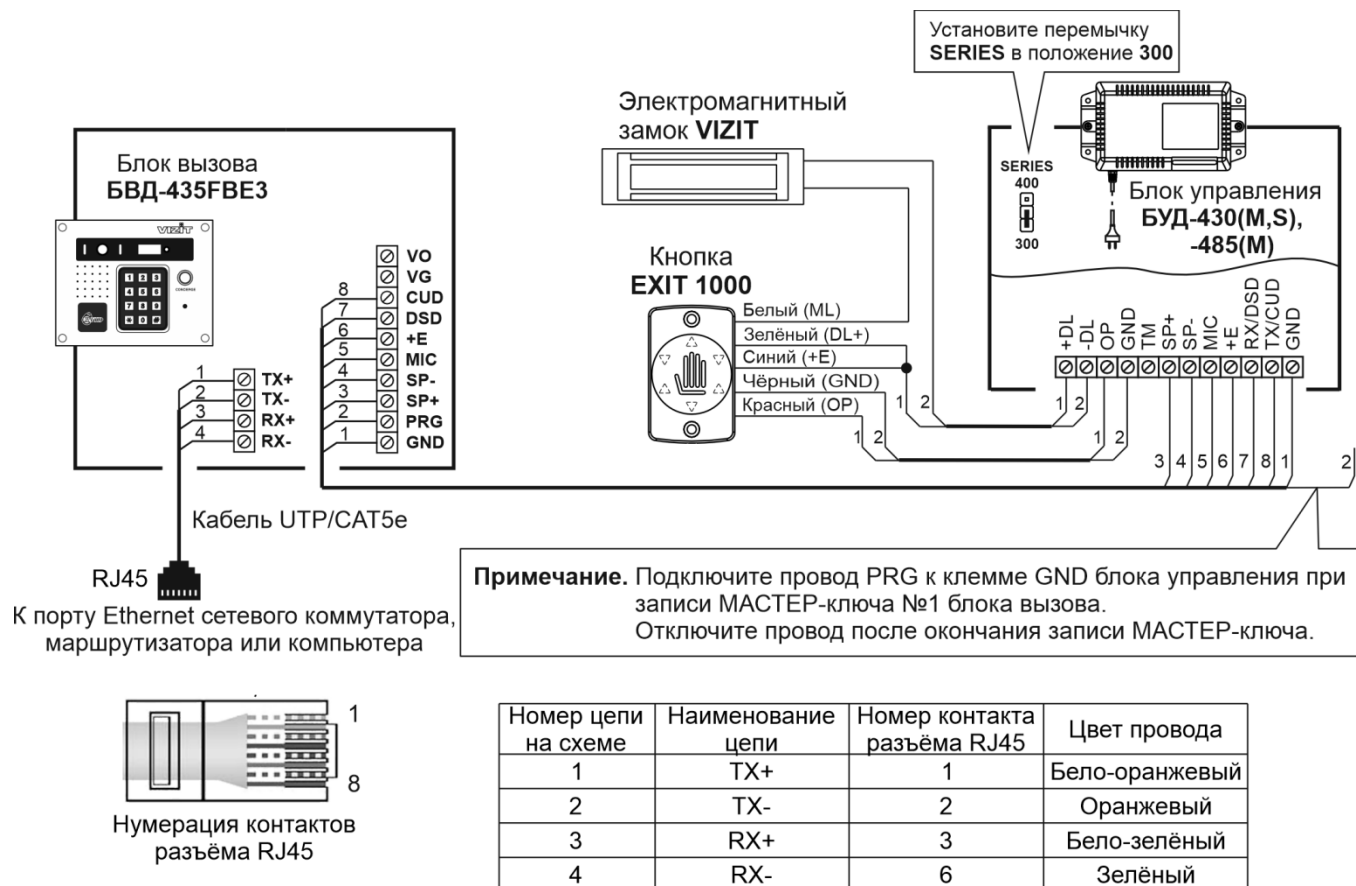
Рисунок 8.1 – Схема соединений блока вызова с блоком управления БУД-430(М,С), -485(М,Р), электромагнитным замком VIZIT-ML400 и кнопкой EXIT 1000
