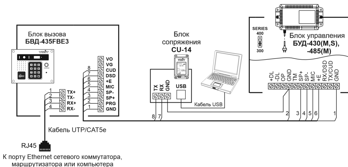
Рисунок 16.1 - Схема соединений блока вызова с блоками управления БУД-430(S, М), -485(М) и блоком сопряжения CU-14
