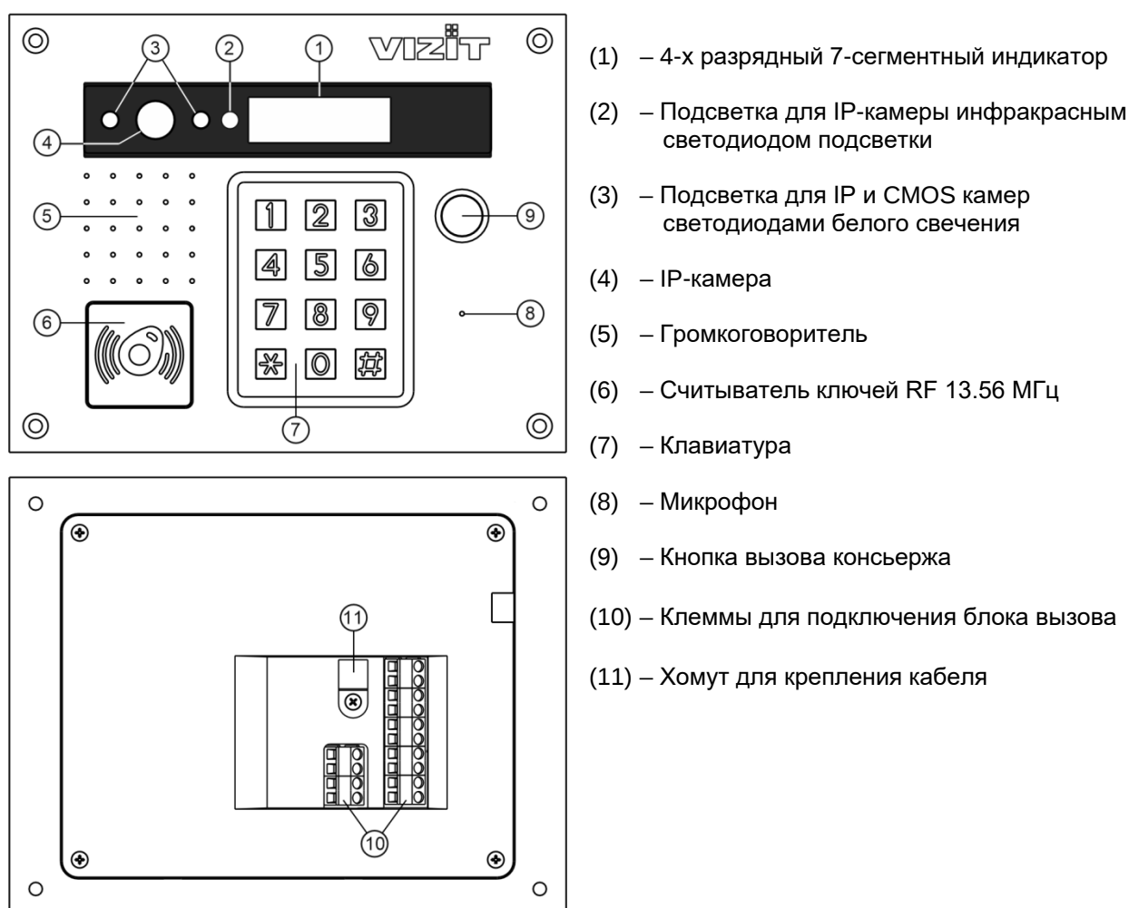
Рисунок 2.1 - Внешний вид блока вызова
