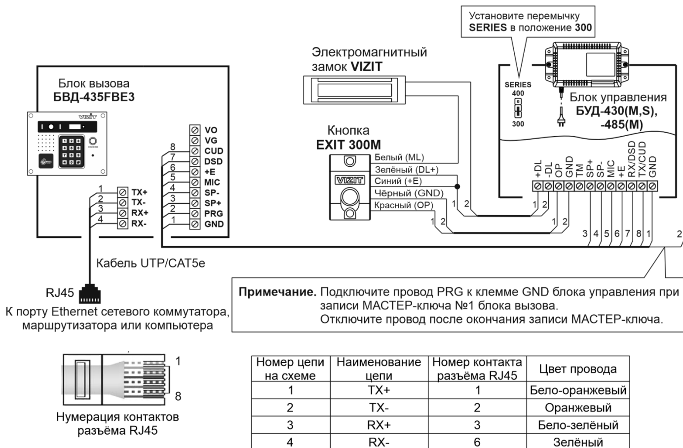
Рисунок 8.3 – Схема соединений блока вызова с блоком управления БУД-430(М,С), -485(М,Р), электромагнитным замком VIZIT и кнопкой EXIT 300M
