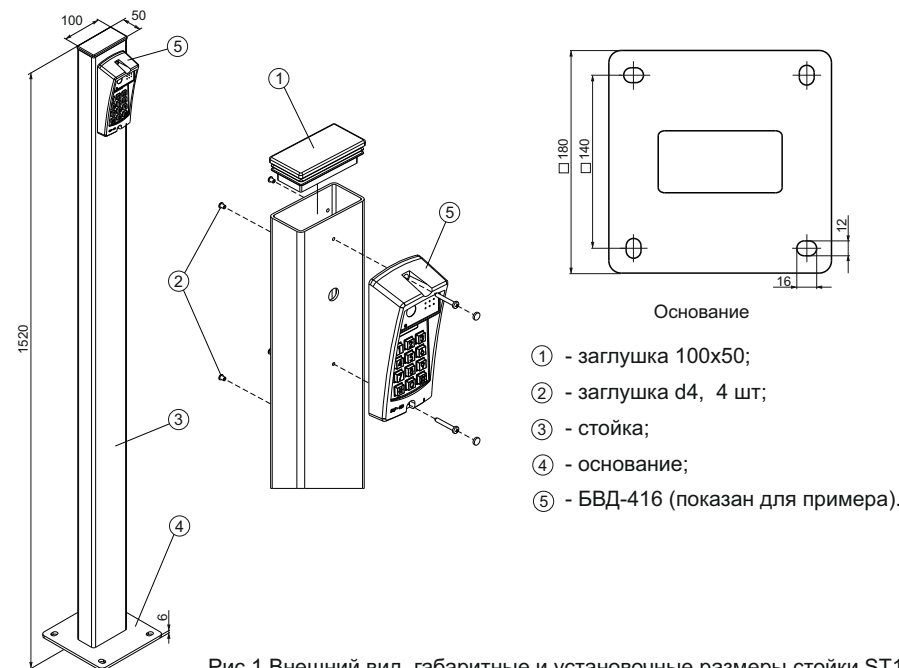
Рис.1 Внешний вид, габаритные и установочные размеры стойки ST10-1
