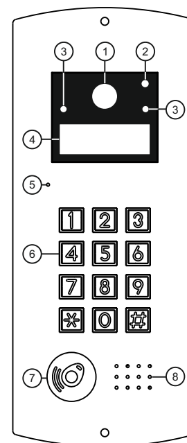
Внешний вид блока вызова
