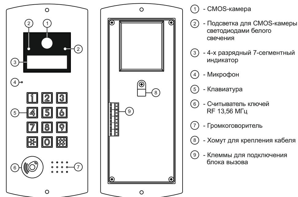
Внешний вид блока вызова
