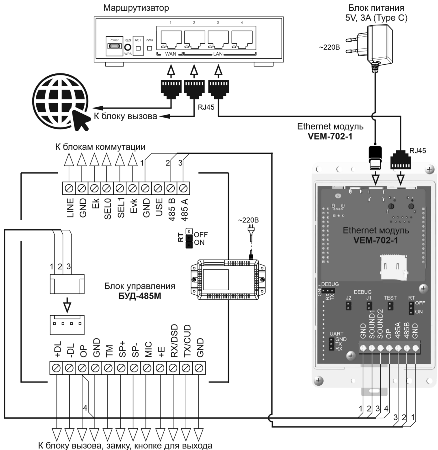
Схема соединений в составе комбинированного (аналогового + IP) видеодомофона. 1 вход: VEM-702-1 + БУД-485М + блок вызова серии 400 или 300.
