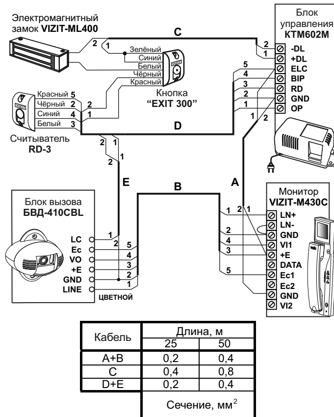
Рисунок 8 - Схема соединений БВД-410СВЛ с блоком управления КТМ602М, считывателем RD-3, монитором VIZIT-M430C, электромагнитным замком VIZIT-ML400 и кнопкой "EXIT 300"
