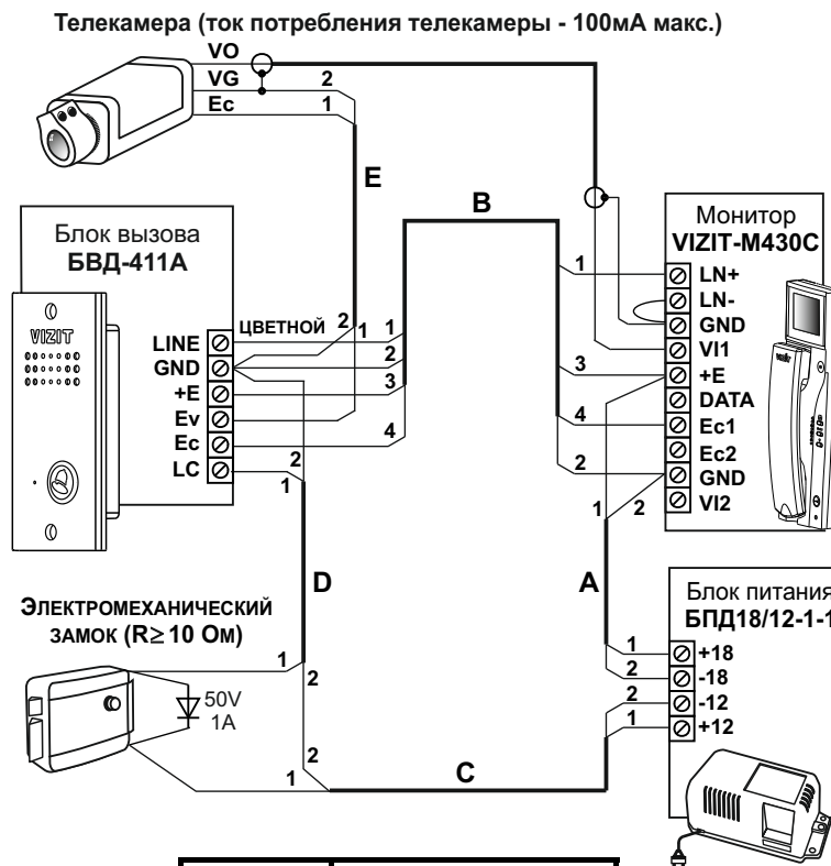
Рисунок 8 - Схема соединений БД-411СВЛ с монитором VIZIT-M402S(C, M, CM) и электромеханическим замком
