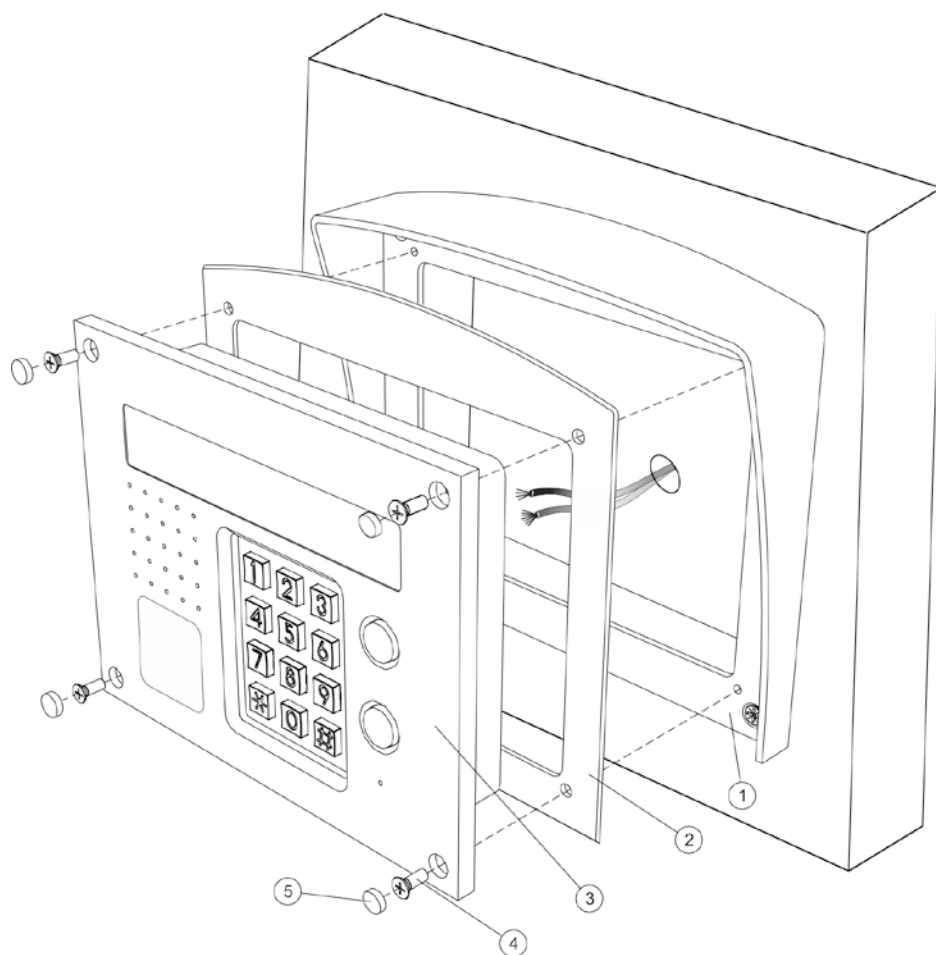
Рисунок 6.3 - Установка блока вызова на монтажный комплект МК-432
