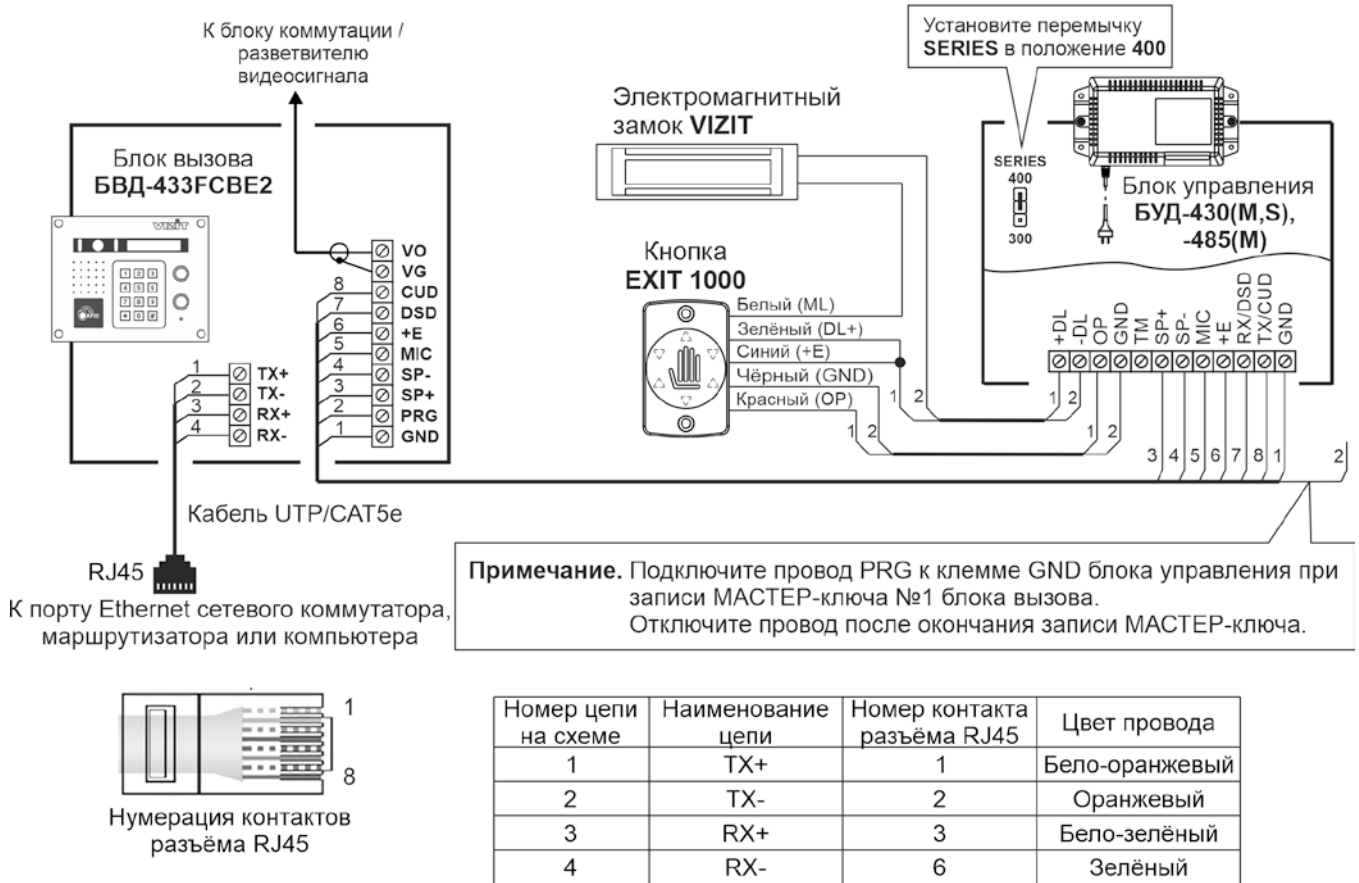
Рисунок 8.1 – Схема соединений блока вызова БВД-433FCBE2 с блоком управления БУД-430(М,С), -485(М), электромагнитным замком VIZIT-ML400 и кнопкой EXIT 1000
