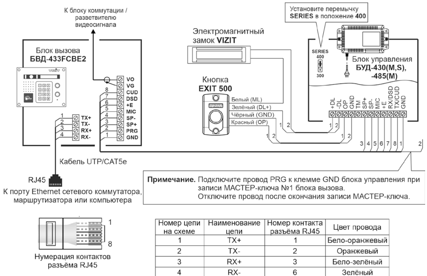
Рисунок 8.2 – Схема соединений блока вызова БВД-433FCBE2 с блоком управления БУД-430(М,С), -485(М,МР), электромагнитным замком VIZIT-ML400 и кнопкой EXIT 500
