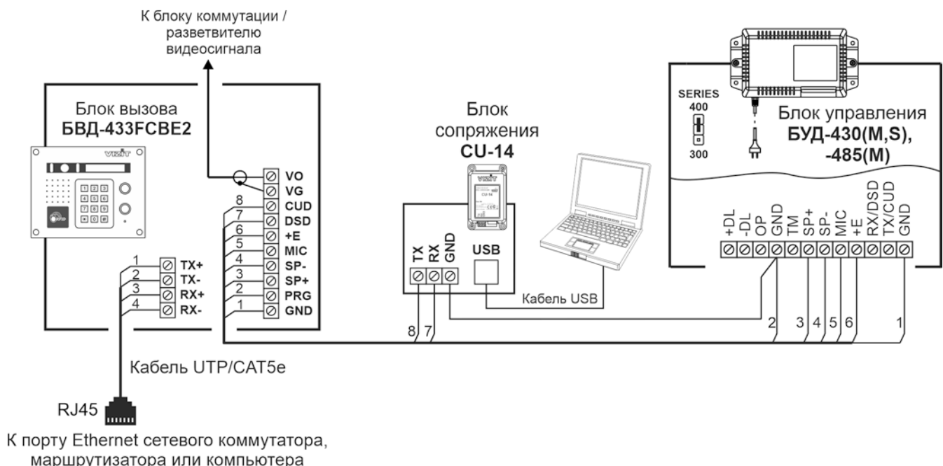
Рисунок 16.1 - Схема соединений блока вызова с блоками управления БУД-430(С, М), -485(М) и блоком сопряжения CU-14
