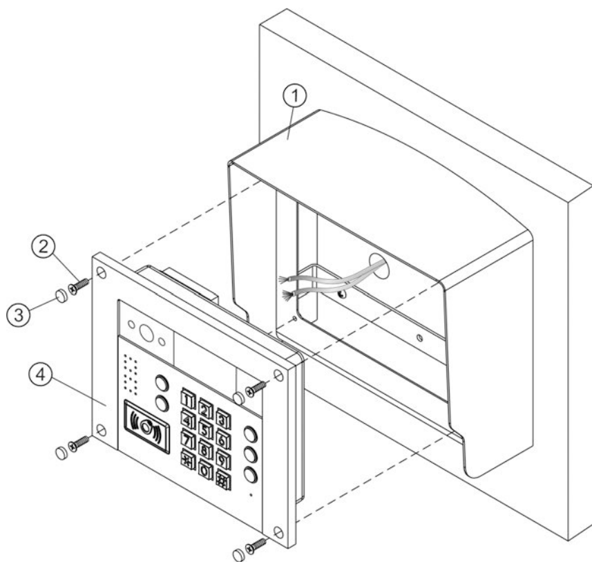
Рисунок 7.4 - Установка блока на монтажный комплект МКФ-432
