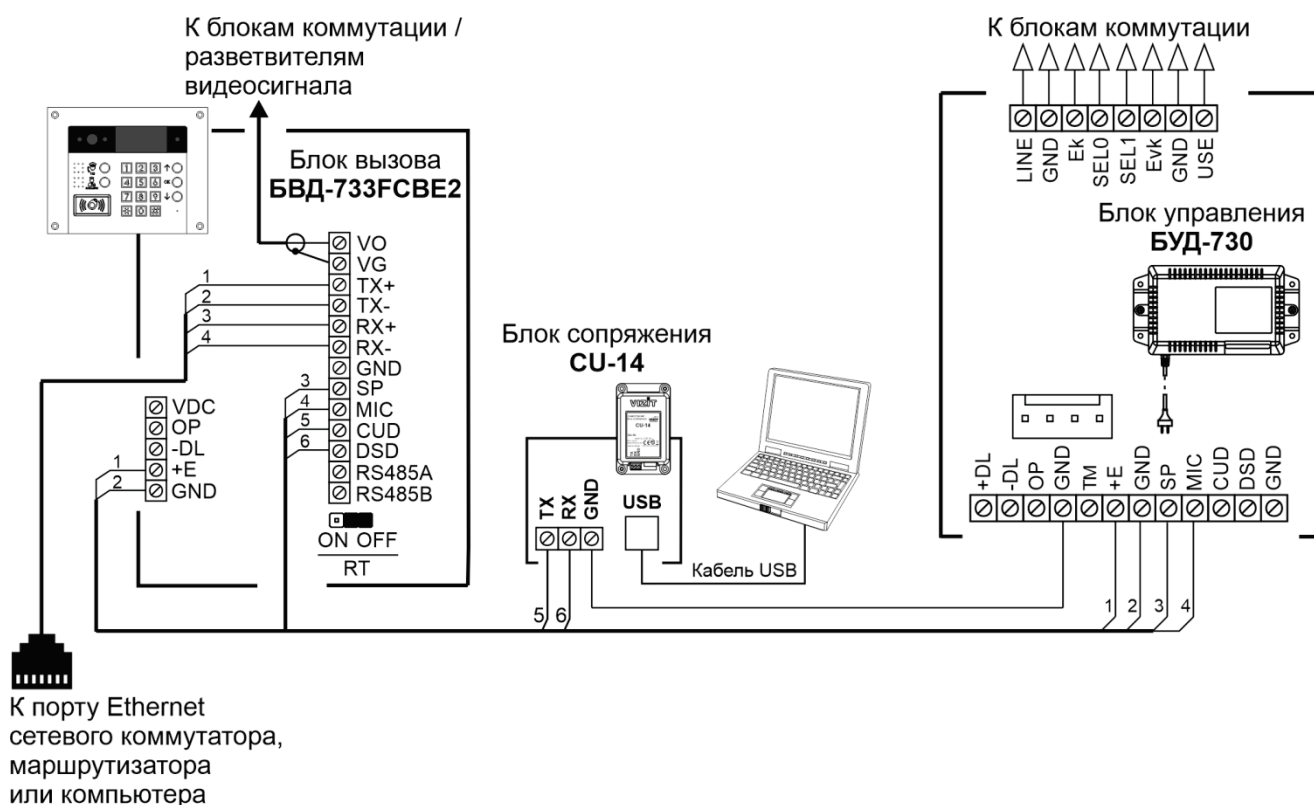
Рисунок 17.1 - Схема соединений блока вызова с блоком управления БУД-730 и блоком сопряжения CU-14
