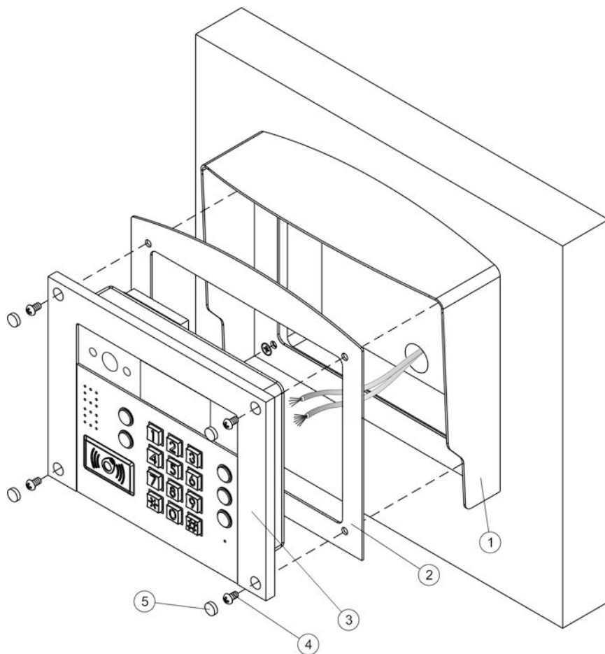
Рисунок 7.3 - Установка блока вызова на монтажный комплект МК-432
