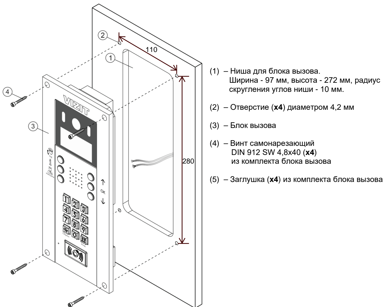
Рисунок 7.2 - Крепление блока вызова на неподвижную часть металлической двери
