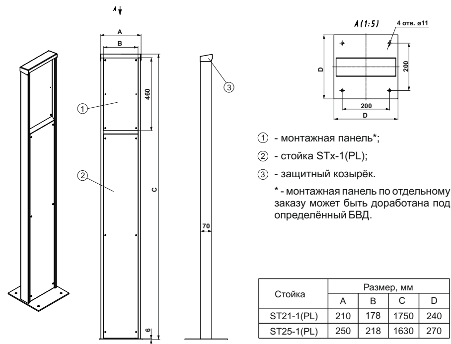
Рис.1 Внешний вид, габаритные и установочные размеры стойки STx-1(PL)
