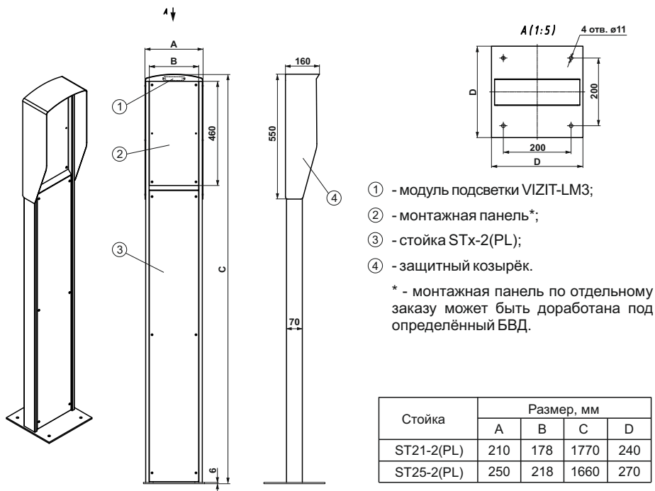
Рис.2 Внешний вид, габаритные и установочные размеры стойки STx-2(PL)
