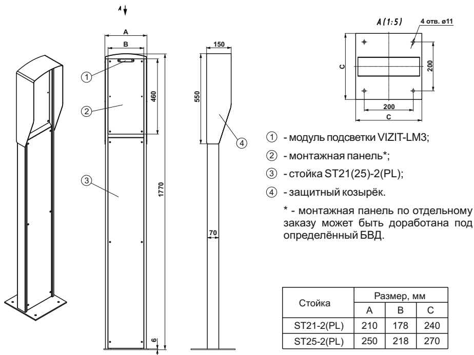
Рис.2 Внешний вид, габаритные и установочные размеры стойки ST21(25)-2(PL)
