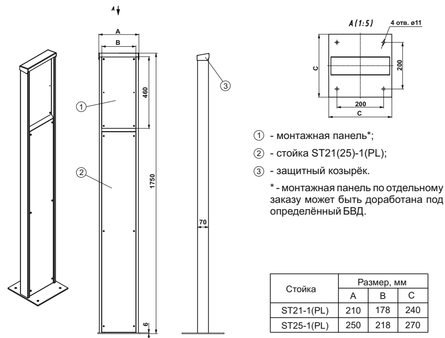
Рис.1 Внешний вид, габаритные и установочные размеры стойки ST21(25)-1(PL)
