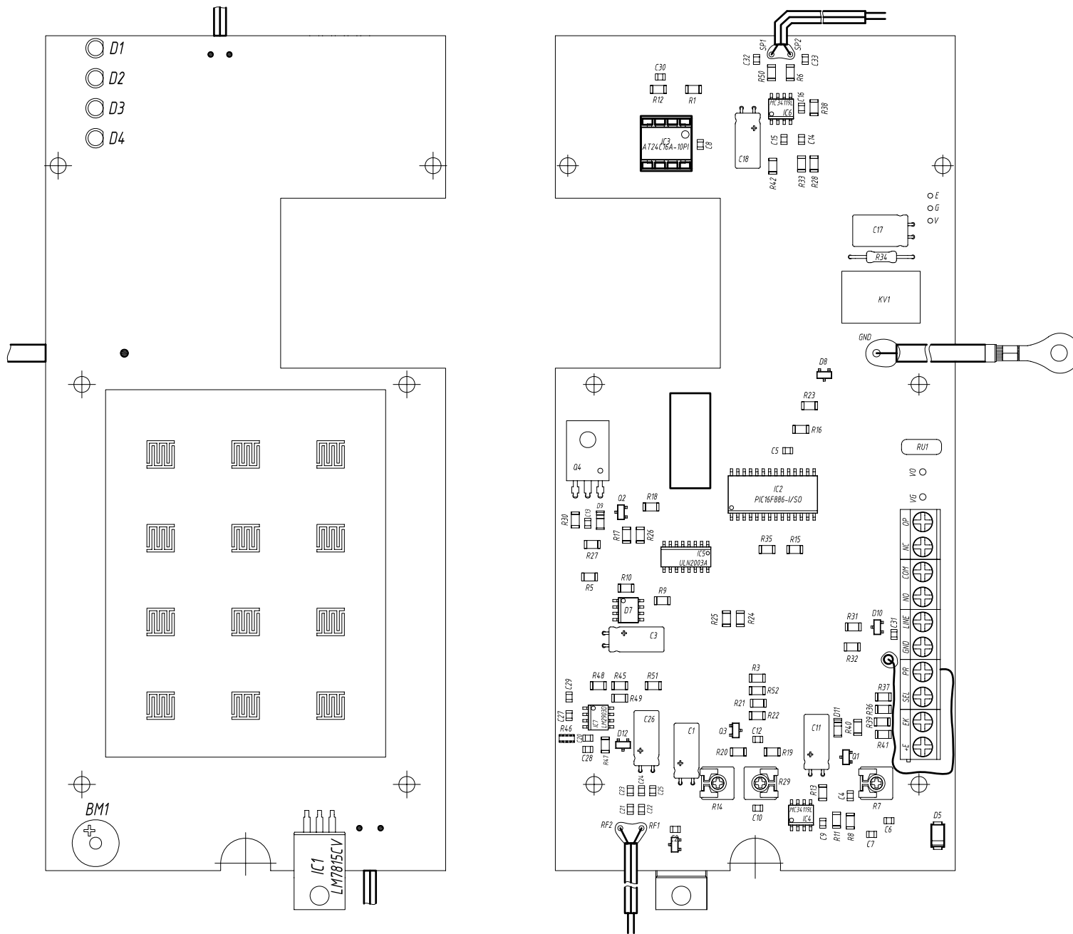
Плата БВД-Н100R Сборочный чертеж
