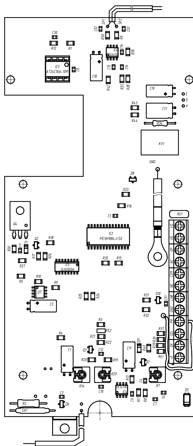
БВД-М100СР Сборочный чертеж
