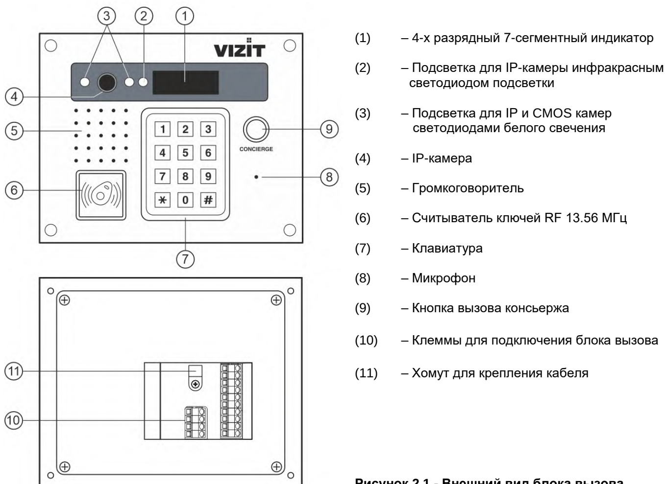
Рисунок 2.1 - Внешний вид блока вызова
