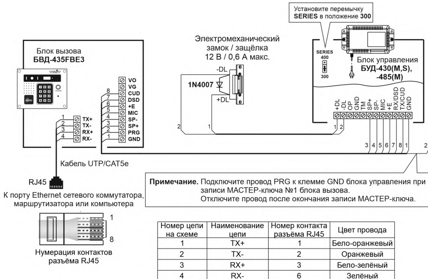
Рисунок 8.4 – Схема соединений блока вызова с блоком управления БУД-430(М,С), -480(С), -485(М,Р) и электромеханическим замком / защёлкой
