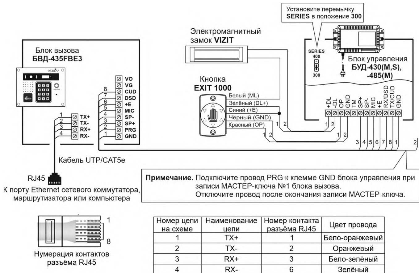
Рисунок 8.1 – Схема соединений блока вызова с блоком управления БУД-430(М,С), -480(С), -485(М,Р), электромагнитным замком VIZIT-ML400 и кнопкой EXIT 1000
