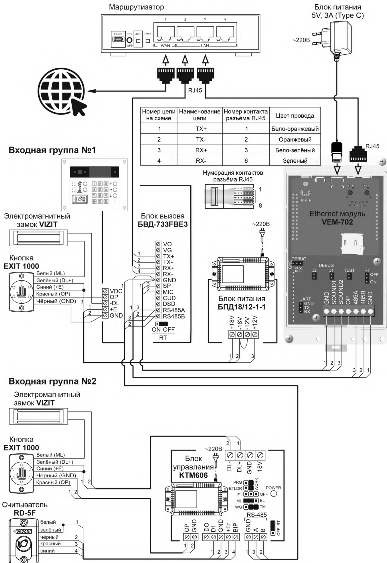
Схема соединений в составе IP видеодомофона. 2 входа: VEM-702 + БВД-733FBE3 + БПД18/12-1-1 + КТМ606.
