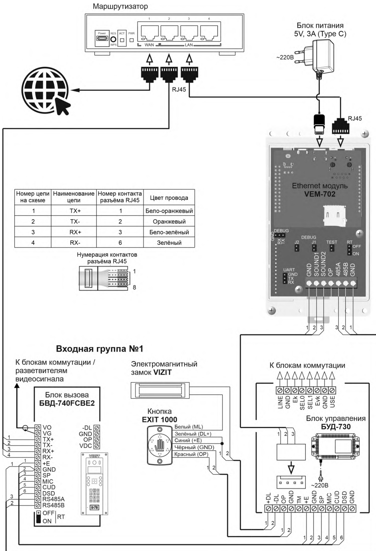
Схема соединений в составе комбинированного (аналогового + IP) видеодомофона. 1 вход: VEM-702 + БВД-740FCBE2 + БУД-730.
