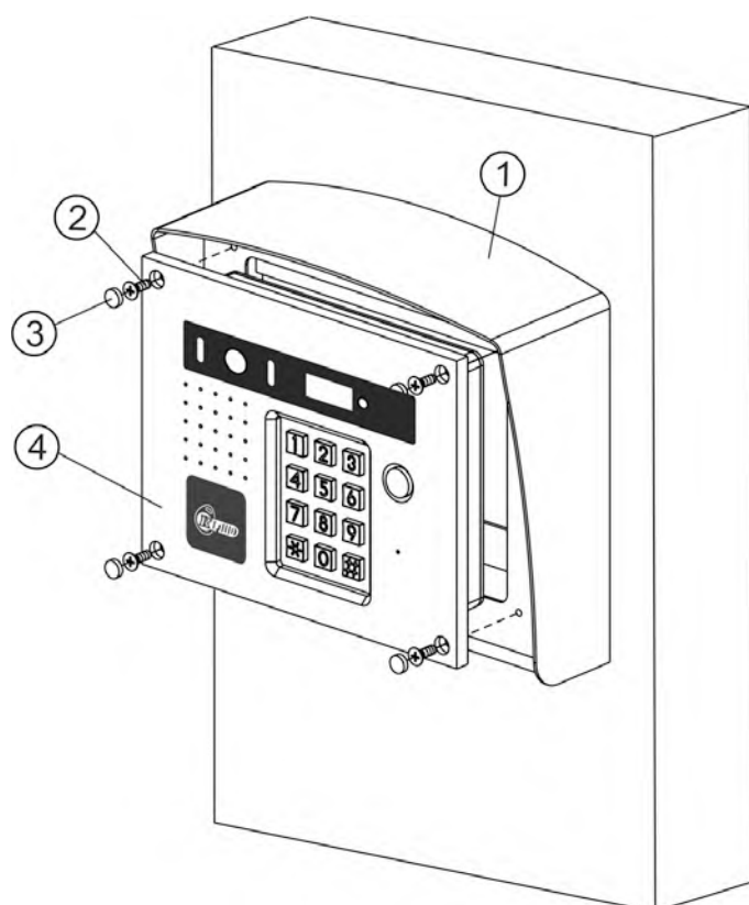
Рисунок 6.5 - Установка блока на монтажный комплект МКФ-432
