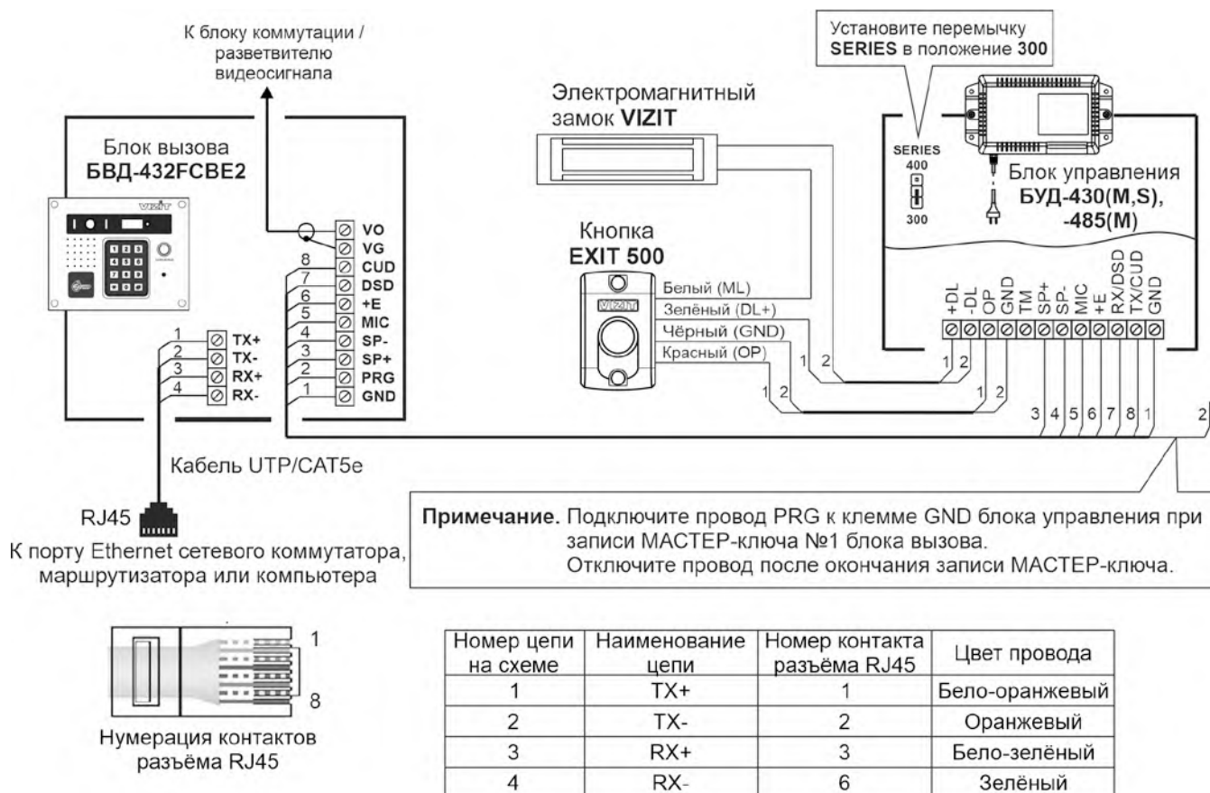
Рисунок 8.2 – Схема соединений блока вызова с блоком управления БУД-430(M,S), -480(S), -485(M,MP), электромагнитным замком VIZIT и кнопкой EXIT 500
