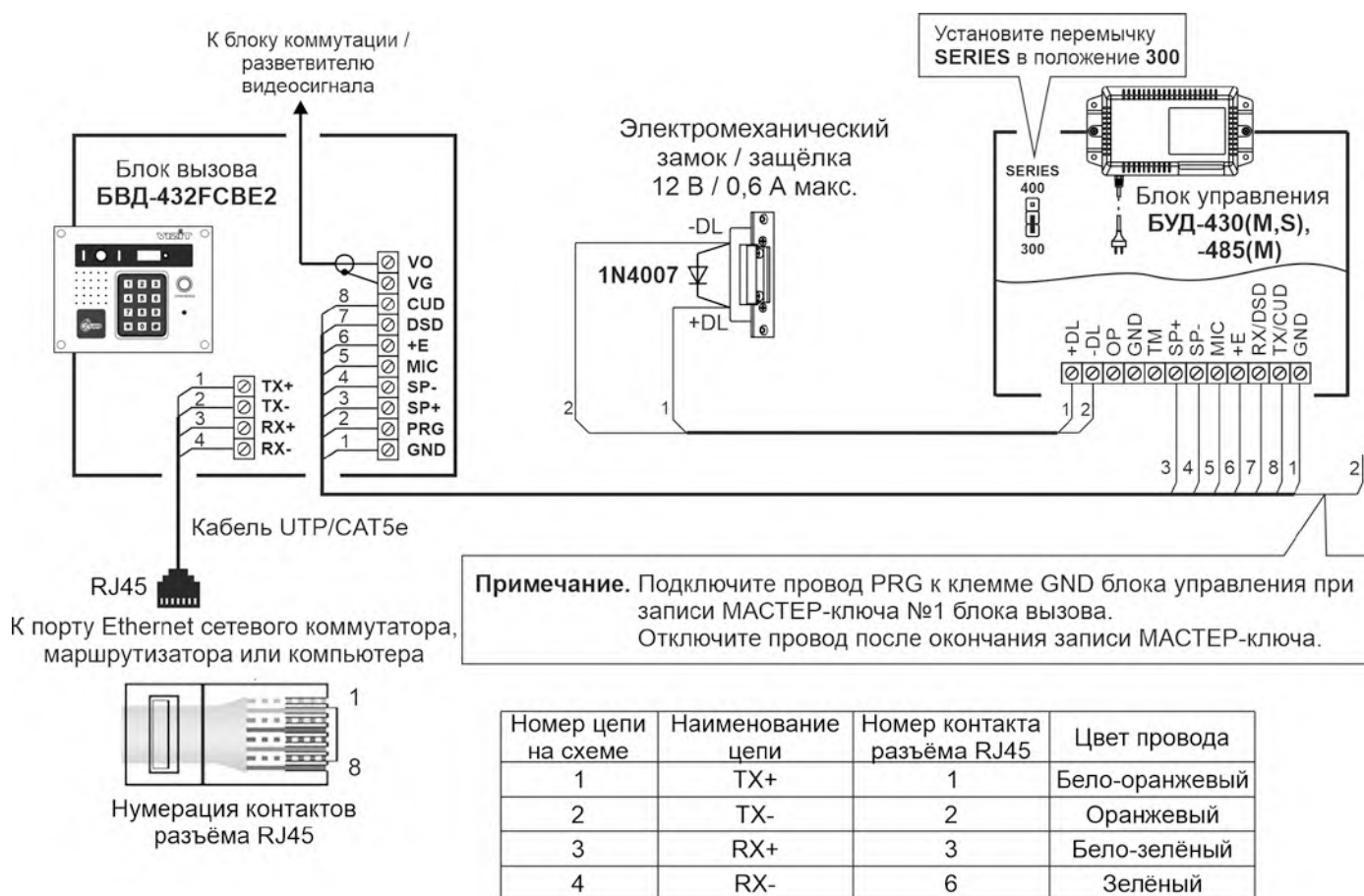
Рисунок 8.4 – Схема соединений блока вызова с блоком управления БУД-430(М,С), -480(С), -485(М) и электромеханическим замком / защёлкой
