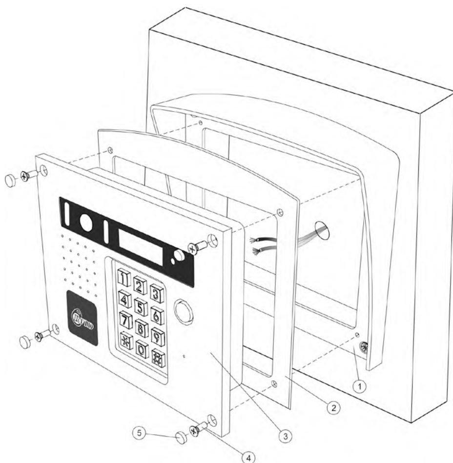
Рисунок 6.4 - Установка блока вызова на монтажный комплект МК-432
