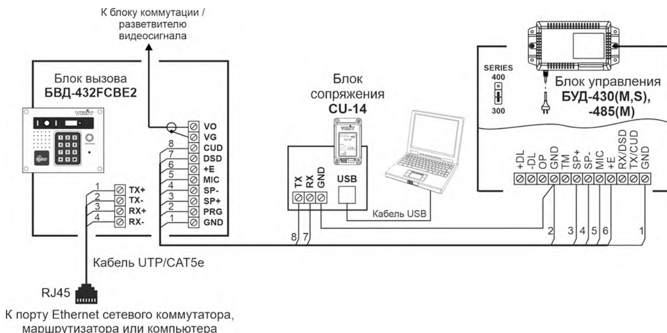
Рисунок 16.1 - Схема соединений блока вызова с блоками управления БУД-430(С, М), -480(С), -485(М) и блоком сопряжения CU-14
