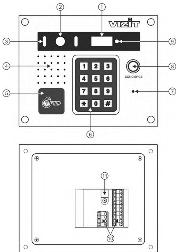
Рисунок 2.1 - Внешний вид блока вызова
