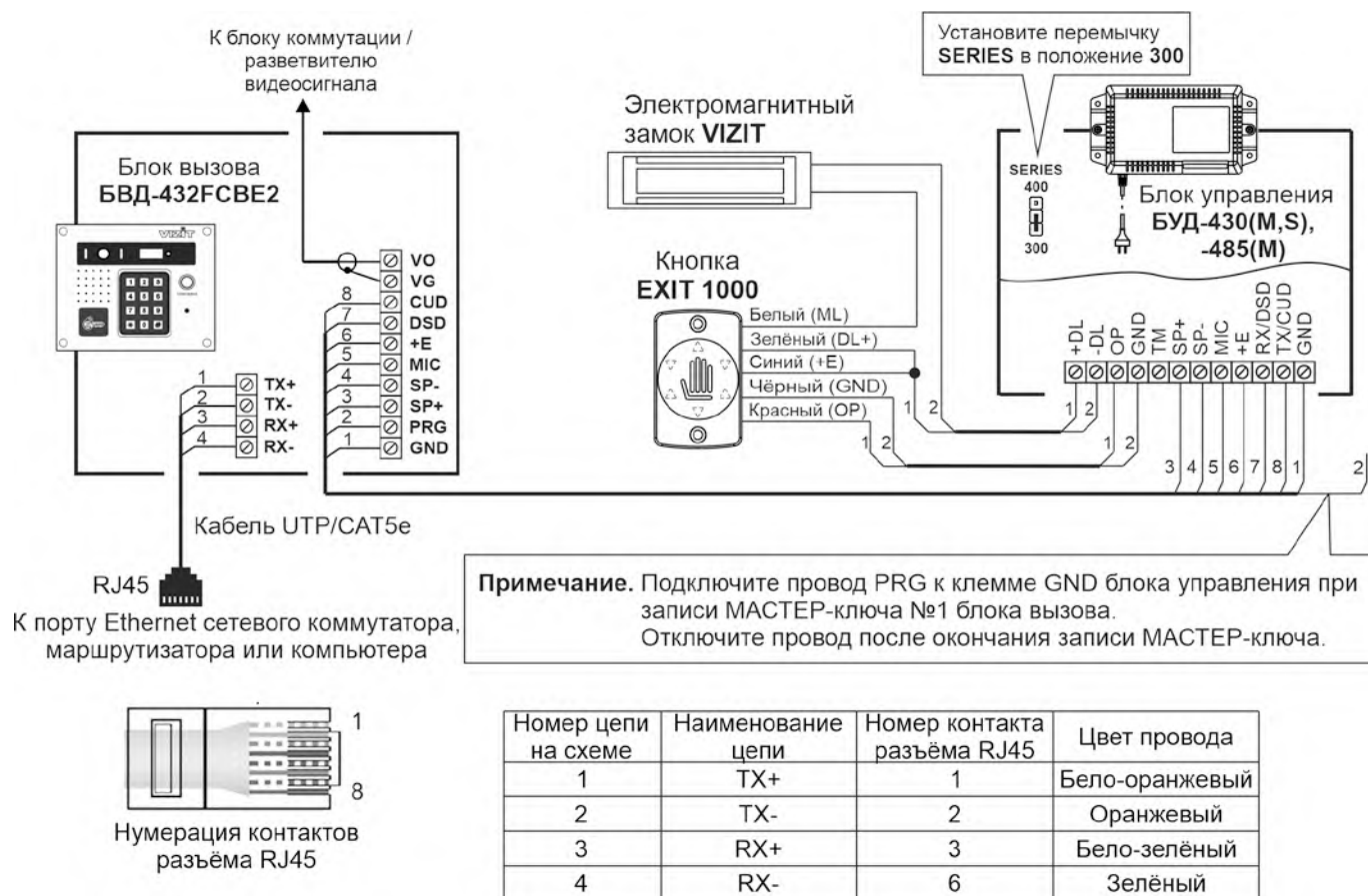
Рисунок 8.1 – Схема соединений блока вызова с блоком управления БУД-430(M,S), -480(S), -485(M), электромагнитным замком VIZIT и кнопкой EXIT 1000
