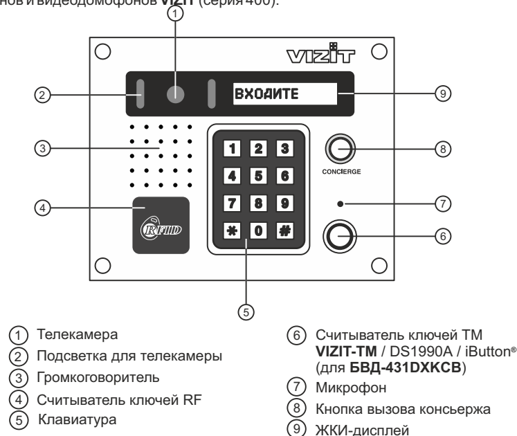
Рисунок 1 - Внешний вид и органы управления блока
