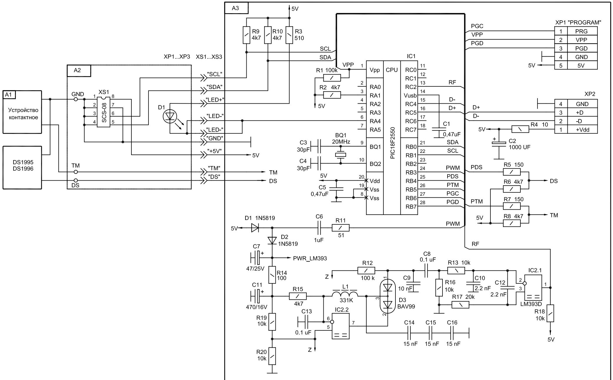
Программатор VIZIT-DM08 Схема электрическая принципиальная
