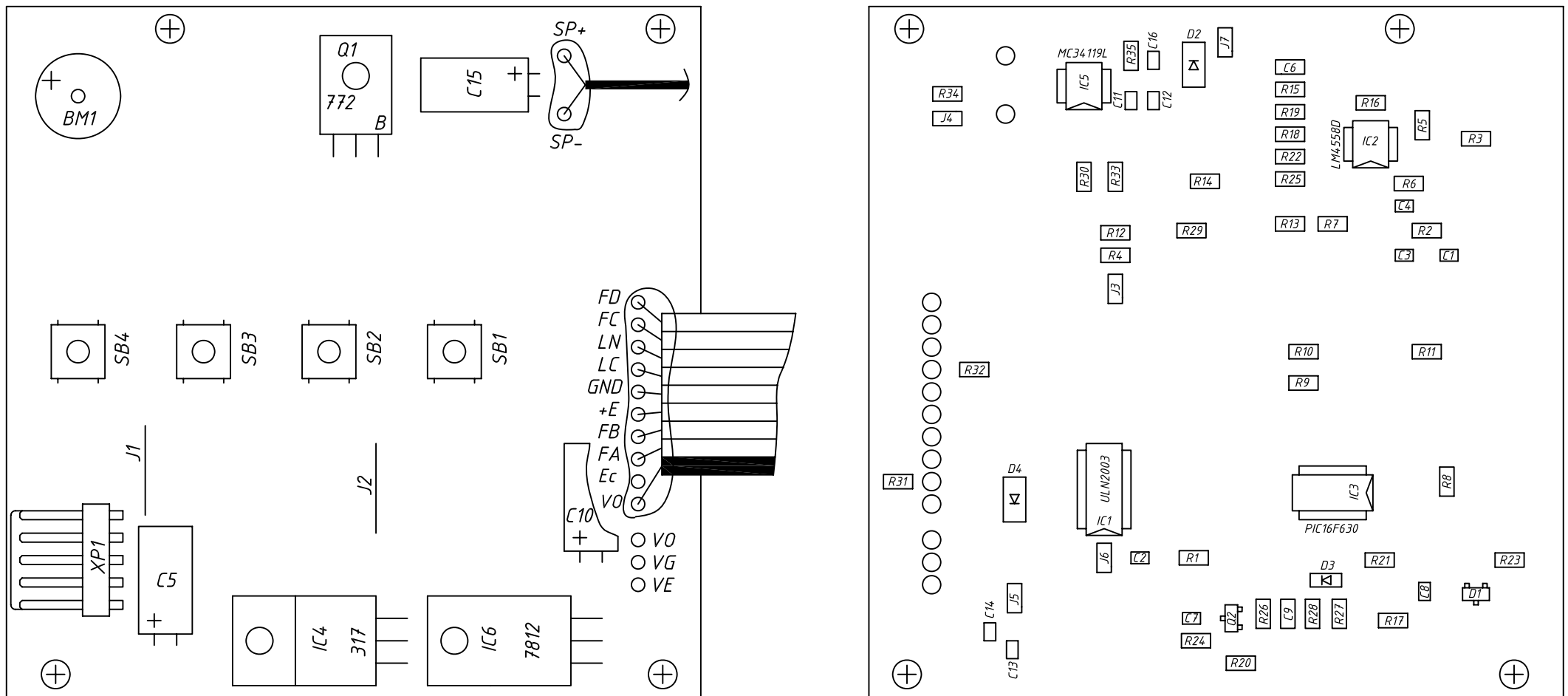
Плата БВД-404СП-4 Сборочный чертеж
