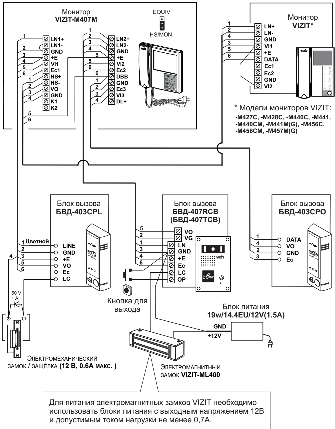
Рисунок 9 - Схема соединений монитора VIZIT-M407M с блоками вызова, дополнительным монитором, электромагнитным и электромеханическим замками
