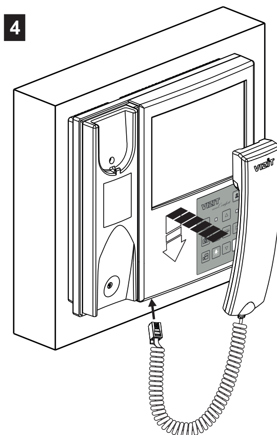
Рисунок 3 - Установка монитора
