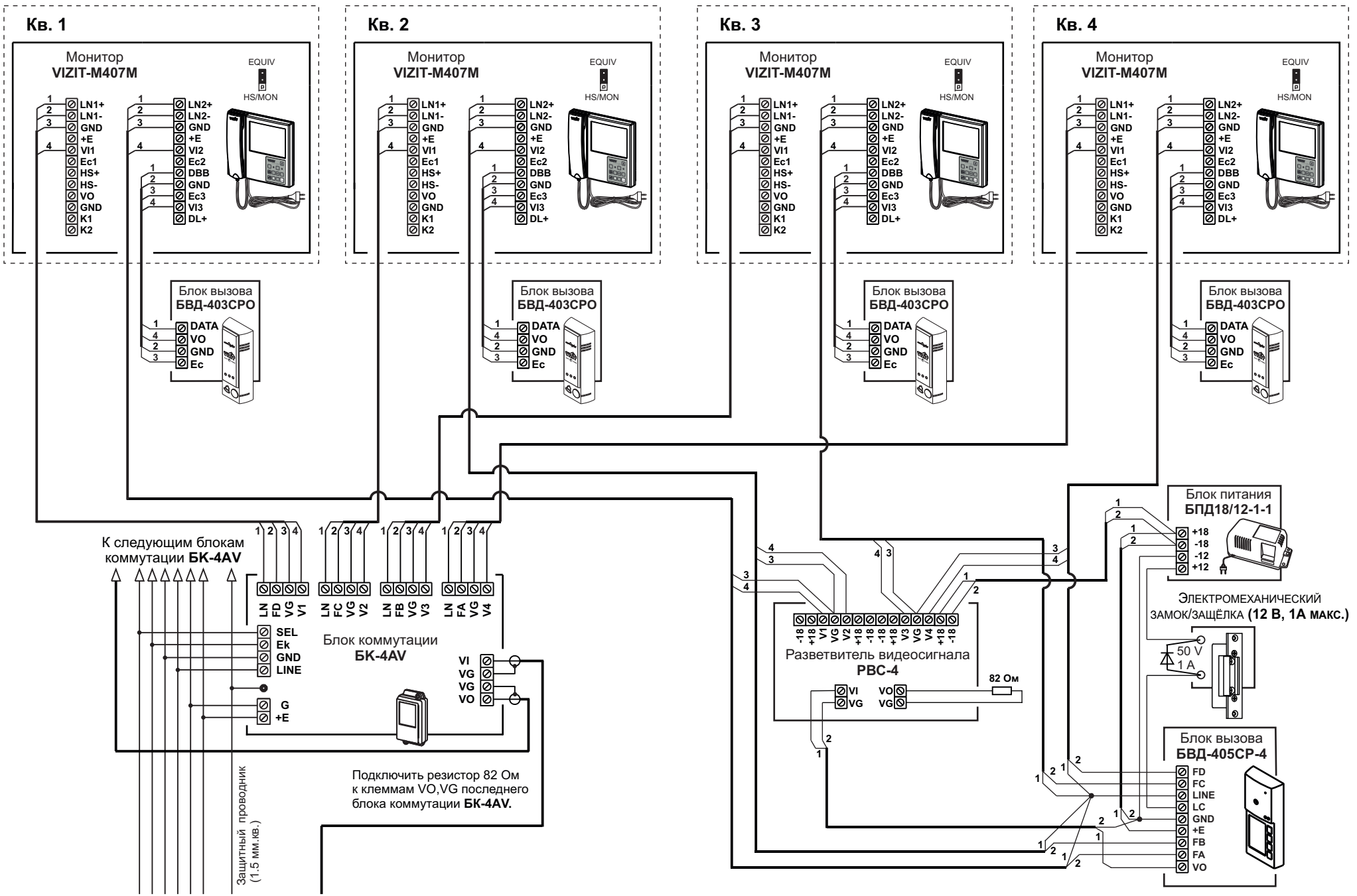
Рисунок 10 - Схема соединений мониторов VIZIT-M407M с блоком коммутации БК-4AV и блоком вызова БВД-405СР-4
