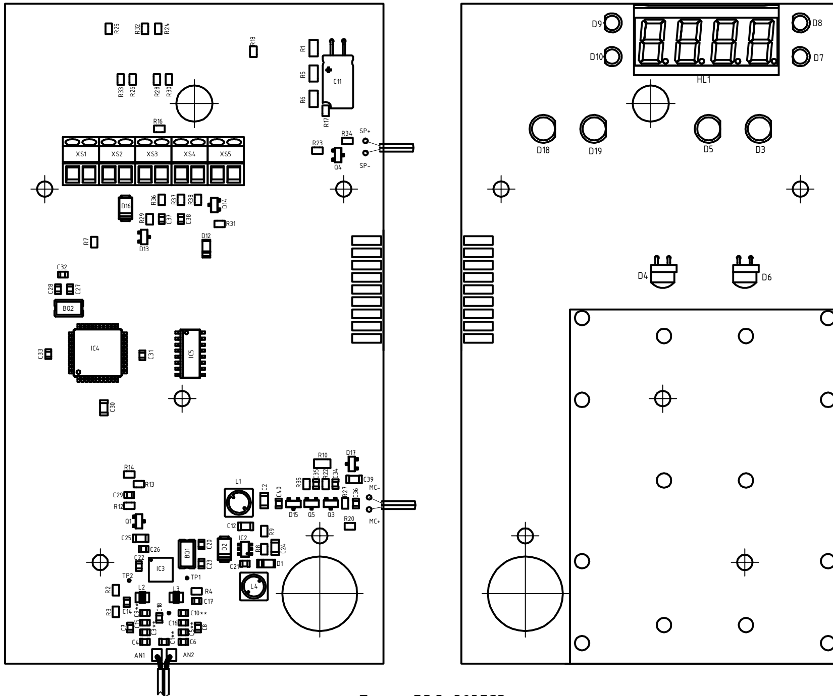
Плата БВД-323FCР Сборочный чертеж
